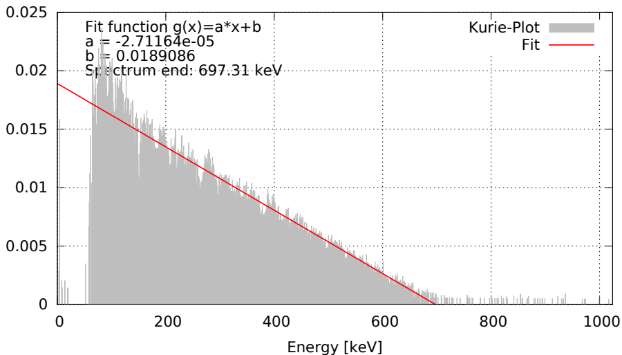
Kurie-Plot zur Endpunktsbestimmung der Elektronenenergie von Sr 90
