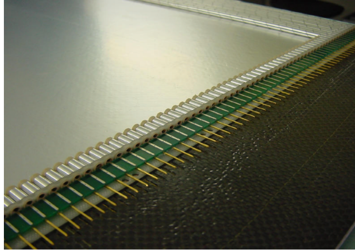
Abbildung 2.4: Ein offenes Endstück, voll bestückt mit allen Röhrcchen, auf die die Strawtubes gesteckt werden sollen. Die Platine mit den Lötstellen für die Anodendrähte und den Kontaktstiften ist bereits eingeklebt.
