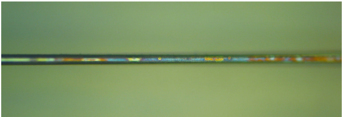
Abbildung 7.18: Bestrahlter Bereich des Anodendrahtes aus Kanal 3b. Die Verfärbungen auf der Drahtoberfläche sind charakteristisch für die bestrahlten Anodendrahte aus Doppelkammer 3.
