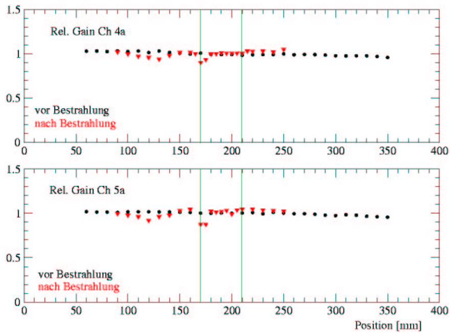
Abbildung 6.14: Die relative Gasverstärkung entlang der bestrahlten Straw-tubes bei 500 ppm Wasser in Ar/CO 2 , vor und nach der Bestrahlung. Die bestrahlte Region entlang der Kanäle erstreckt sich über 4 cm von Position 170 bis 210 und ist durch die Linien markiert. Position 0 entspricht dem unteren, Position 400 dem oberen Ende des Moduls. Die Gasflussrichtung war in Richtung Position 400.
