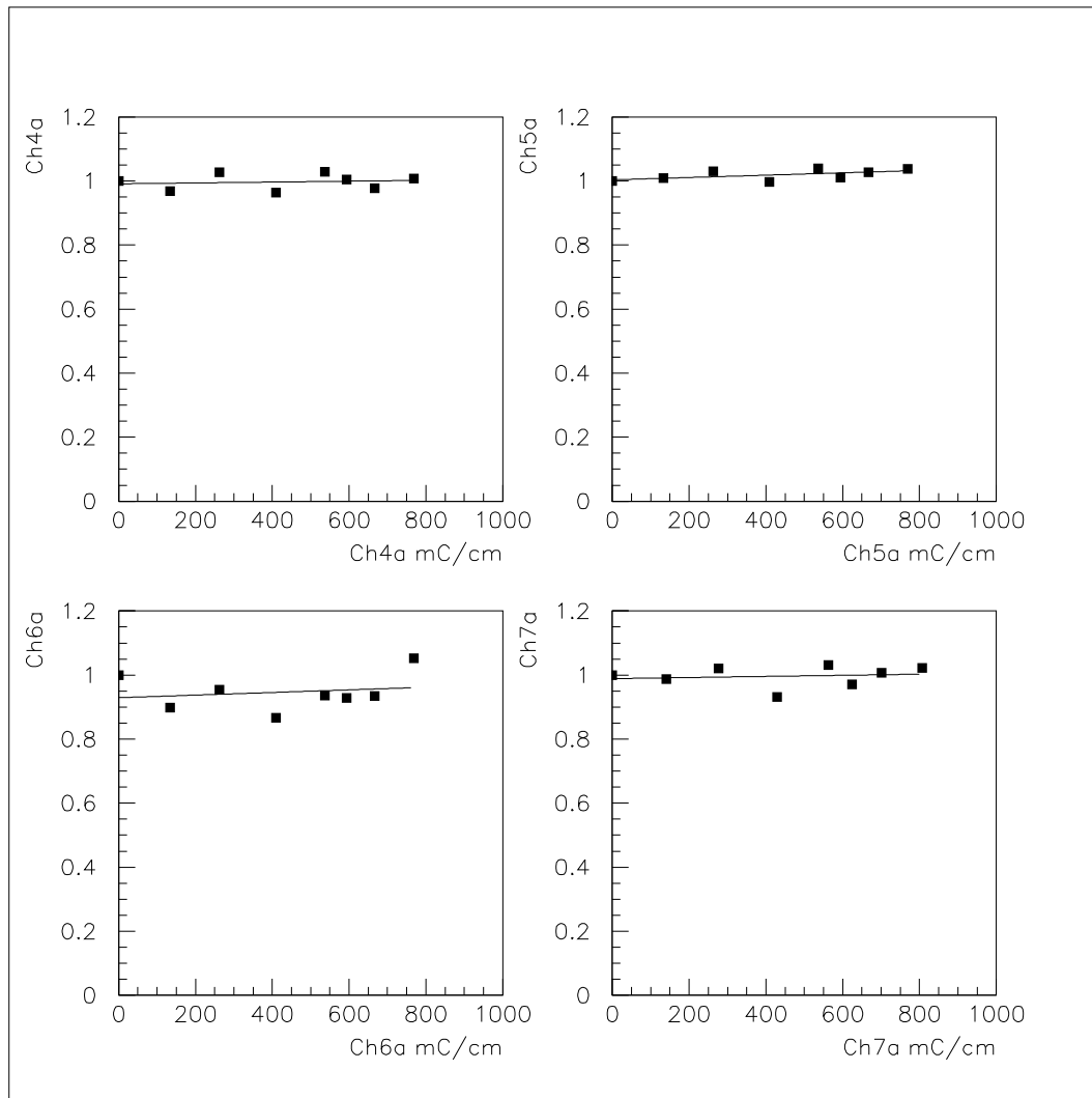
Abbildung 7.4: Die relativen Gasverstärkungen aufgetragen über die angesammelten Ladungen in den Kanälen 4a, 5a (ohne Drahtpositionierern) und 6a, 7a (mit Drahtpositionieren). Die Gasverstärkung wurde jeweils an Position 250 gemessen (Abbildung 7.1). Zählgas war Ar/CO 2 .
