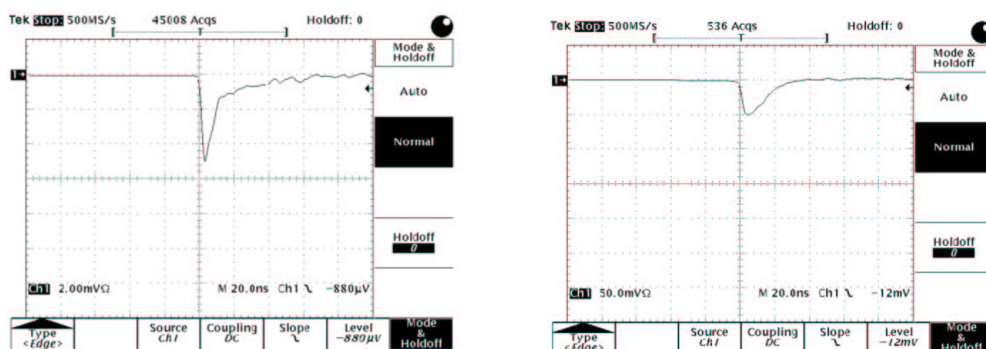
Abbildung 3.8: Signale aus einem Strawtube ohne Vorverstärker. Zählgas war Ar/CO 2 /CF 4 . Links: 55 Fe-Signal bei 1500 V. Die Signalamplitude ist 7 mV. Rechts: Dunkelpuls bei 1500 V. Die Signalamplitude ist 50 mV. [50]
