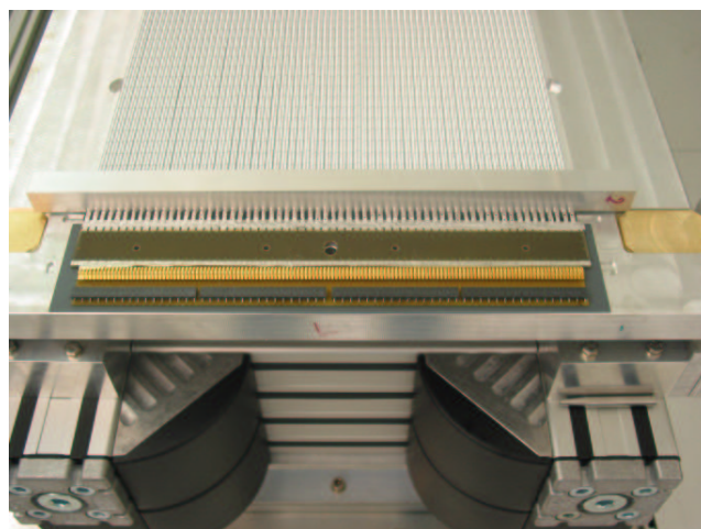
Abbildung 2.25: Die Strawtubes werden ins Template gelegt und angesaugt. An ihren Enden werden sie mit aufgelegten Gegenschablonen zusätzlich in Position gehalten. Die Föhnchen der Strawtubes werden auf einen Kupferstreifen gelötet. Der Streifen wird an die Massenkontakte der HV-Durchführungsplatine gelötet.
