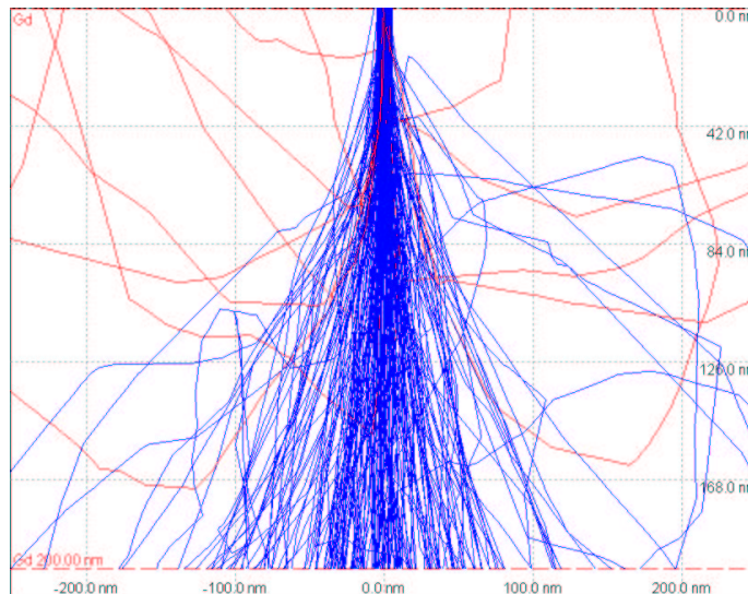
Abbildung 4.7: Von oben trifft ein gebündelter Elektronenstrahl mit 35 keV auf eine 200 nm dicke Gadoliniumschicht. Die roten Trajektorien werden zurückgestreut, die blauen gelangen durch die Folie hindurch. Diese Simulation ist mit dem Programm CASINO durchgeführt worden.
