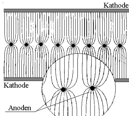
Abbildung 3.3: Aufbau sowie Verlauf der Feldlinien in einer Vieldrahtkammer [Kle00].
