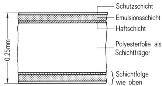
Abbildung 2.5: Aufbau eines beidseitig beschichteten Röntgenfilms [Mor95]. Bei der Erweiterung zum Film-Folien-System wird ein solcher Film zwischen zwei Verstärkungsfolien gebracht. In diesen wird Röntgenstrahlung in sichtbares Licht umgewandelt, das dann in beiden Schichten des Films nachgewiesen wird.
