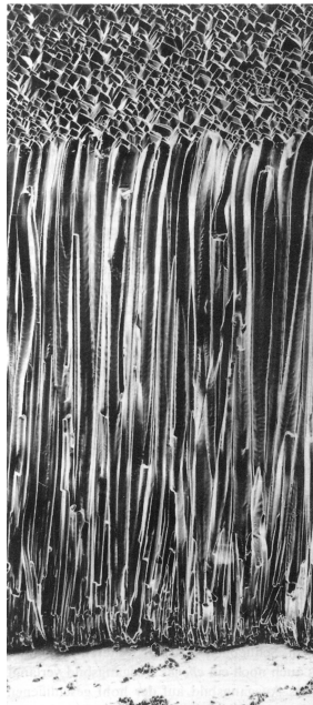
Abbildung 2.12: Säulenförmige Struktur von Cäsiumjodid [Mor95].
