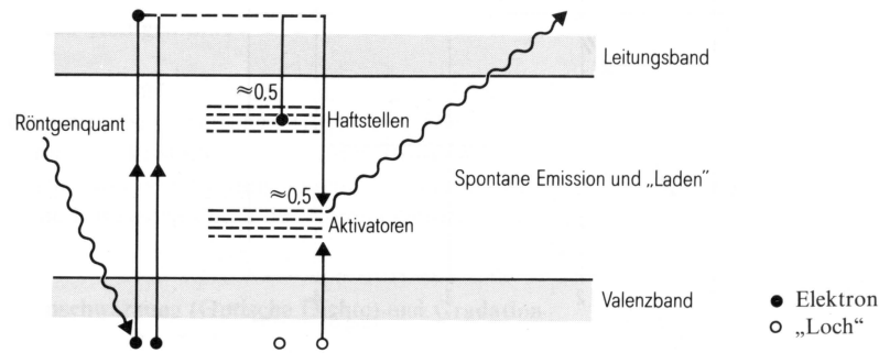
Abbildung 2.8: Belichtungsvorgang (Laden) der Speicherfolie. Die durch die Röntgenstrahlung erzeugten Elektron-Loch-Paare diffundieren durch den Leuchtstoff, bis das Elektron aus dem Leitungsband auf eine Haftstelle trifft und dort gespeichert wird [Mor95].
