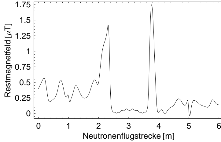
Abbildung 8.3: Das longitudinale Restmagnetfeld innerhalb der \mu -Metall Abschirmung. Die beiden Spitzen befinden sich am Rand der doppelwandig abgeschirmten Arme des RESEDA-Spektrometers.
