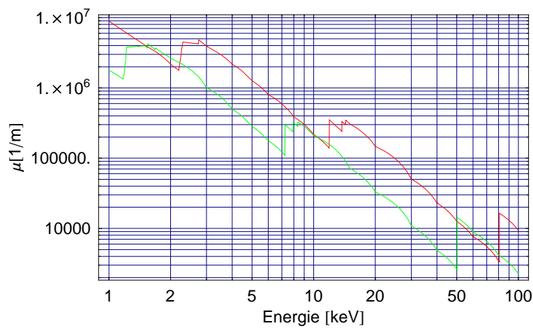
Abbildung 4.3: Absorptionskoeffizient am Beispiel für Gadolinium (grün) und Gold (rot). Im Anhang A.1 ist dieser für Argon, Kapton und Kupfer dargestellt. In Abbildung 5.1 ist dies für weitere Materialien dargestellt.
