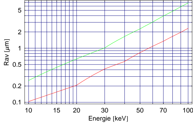
Abbildung 4.9: Reichweite von Elektronen in Festkörpern am Beispiel von Gadolinium (grün) und Gold (rot). Dargestellt ist hier der average reach ( R_{av} ) Wert. Weitere Beispiele sind im Anhang A.2 und in Abbildung 5.2 dargestellt.
