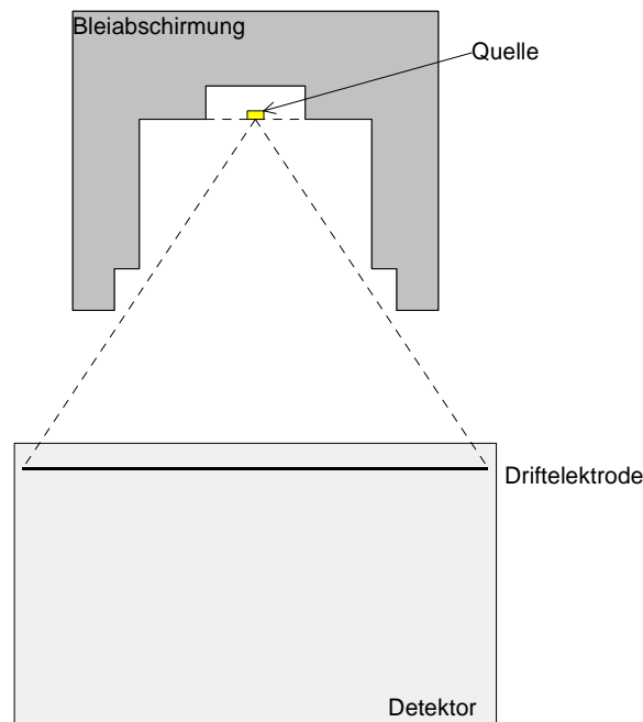
Abbildung 6.6: Draufsicht auf Detektor und Bleiabschirmung der Quellen. Je nachdem, welchen Abstand der Detektor zu der Bleibox hat, muß berücksichtigt werden, daß der Raumwinkel auch durch die Kanten der Bleiabschirmung limitiert sein kann.
