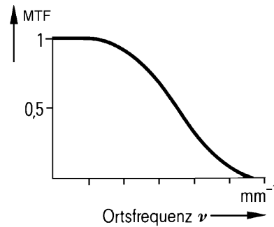
Abbildung 2.3: Typischer Verlauf der Modulationsübertragungsfunktion [Mor95].
