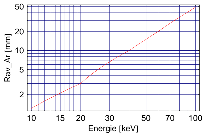
Abbildung A.5: Reichweite von Elektronen in Argon. Dargestellt ist der average reach ( R_{av} ) Wert.
