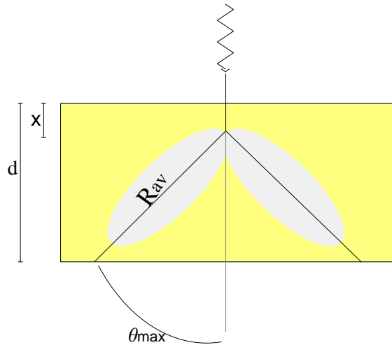
Abbildung 4.6: Darstellung der in der Rechnung verwendeten Abkürzungen in Bezug auf Konversion und Reichweite. Von oben tritt das Photon in die Materieschicht der Dicke d ein (gelb dargestellt) und gelangt bis zur Stelle x , an der es konvertiert wird. Die Wahrscheinlichkeit, in welche Richtung das Photoelektron emittiert wird, ist durch die weiß Keulen veranschaulicht.
