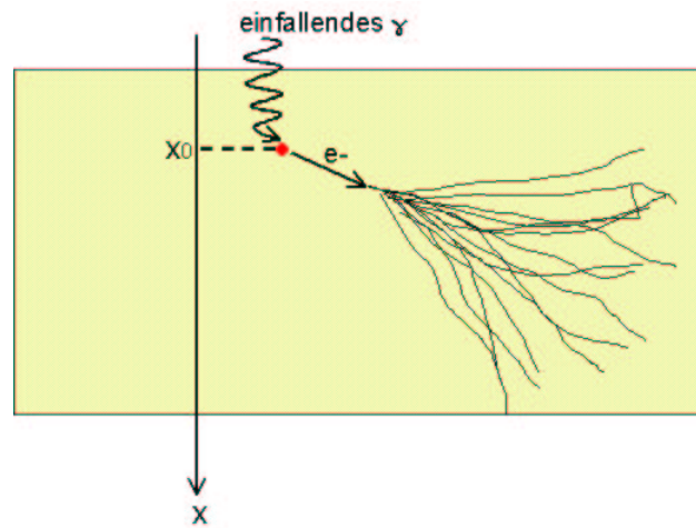
Abbildung 4.2: Schematische Darstellung der Prozesse beim Eindringen eines Photons in Materie. Die vielen verschiedenen Trajektorien zeigen die möglichen Wegstrecken des Elektrons auf.
