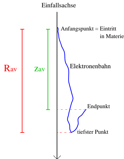
Abbildung 4.8: Schematische Darstellung zur Veranschaulichung der verschiedenen Definitionen der Reichweite von Elektronen in Materie.
