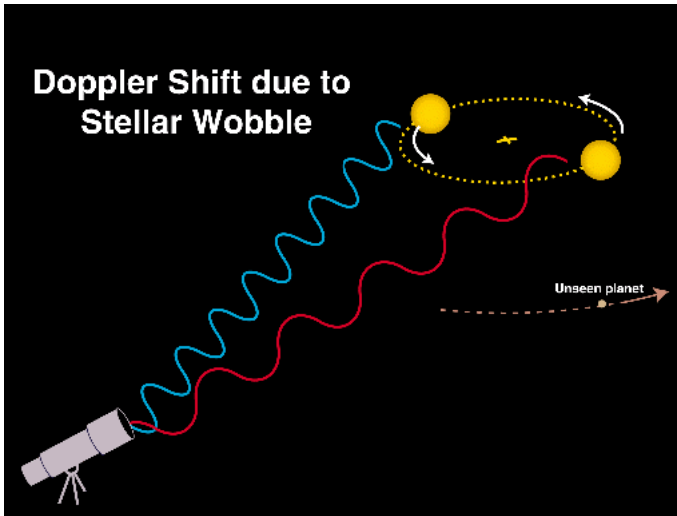
Messprinzip: messe Bewegung der Sonne um den Schwerpunkt
